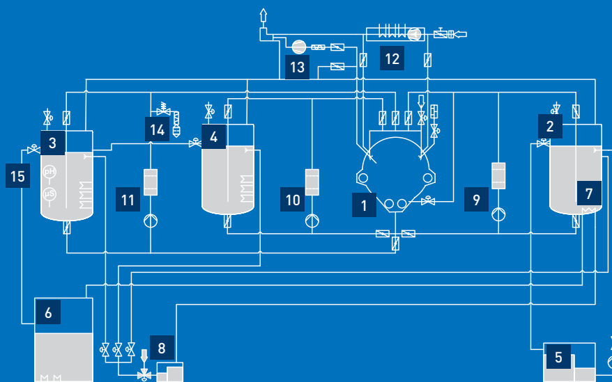
➤ EcoCwave 工艺流程图例 (带蒸馏装置的3槽系统)
